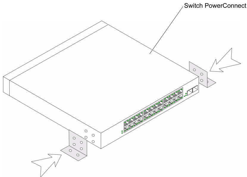
Obrázek 1-2. Instalace držáku při montáži na zeď
